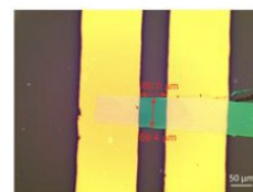
有機半導体
