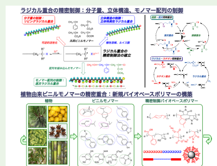
本グループで研究を進めている高分子合成
