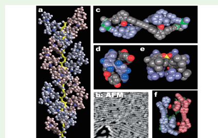
これまでに合成したらせん高分子・超分子 a) ポリフェニルアセチレン、b) ポリイソシアニド、 c) 相補的二重らせん、d) 水溶性二重らせん、 e) ヘリケート、f) 三重らせんシリンドラー
